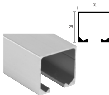
懸吊式軌道 - 上L型
