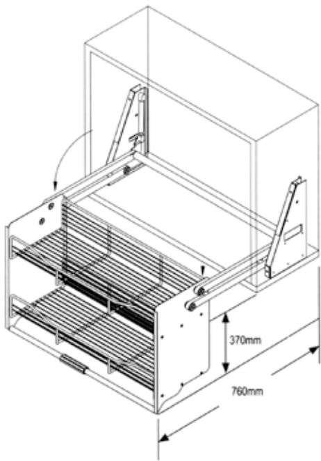
雙緩衝 - 收納升降櫃 - 不鏽鋼
