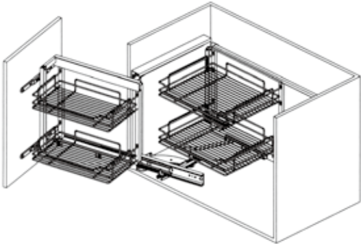
旋轉緩衝小怪物右開 - 鐵鍍鉻
