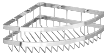
AK-523 貴族型轉角架 規 格 230 x 230 x 90 mm 材 質 不鏽鋼 附件：銅螺帽 x4 只
